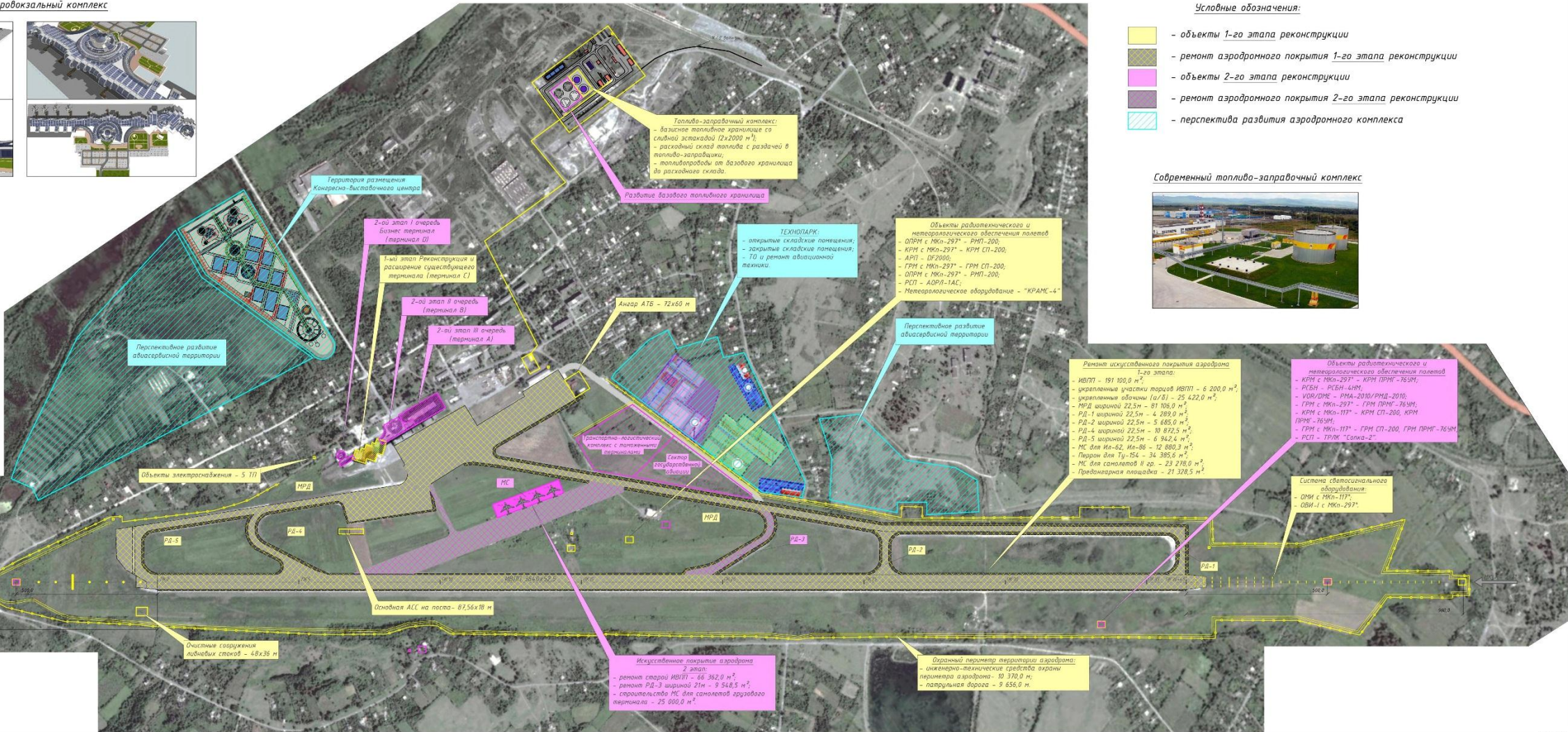
Современный аэровокзальный комплекс
